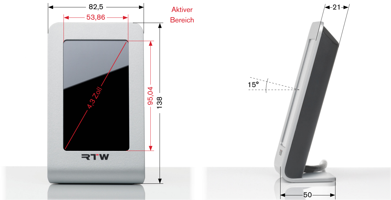
1 | Frontansicht
