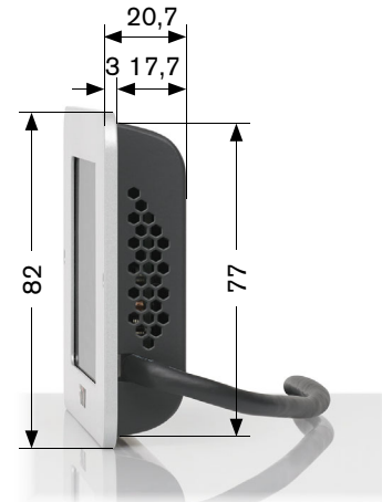
2 | Seitenansicht
