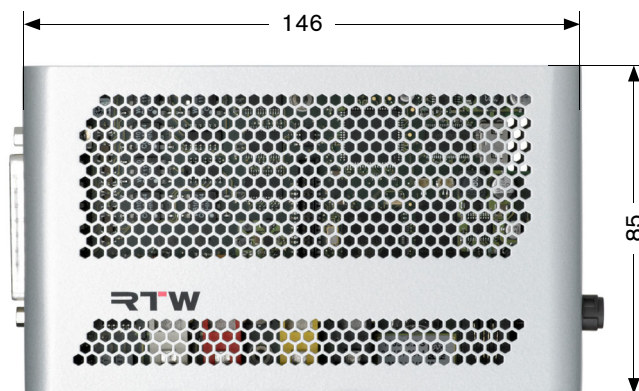
1 | Draufsicht
