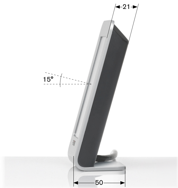
2 | Seitenansicht
