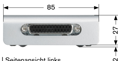
3 | Seitenansicht links
