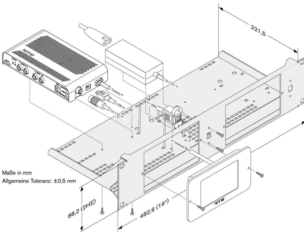
1 | Schematische Darstellung der Montage eines TM3S mit Option TM3-2U in Baugruppenträger TM3-MA2U
