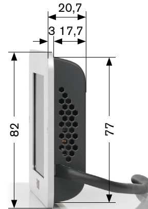
2 | Seitenansicht
